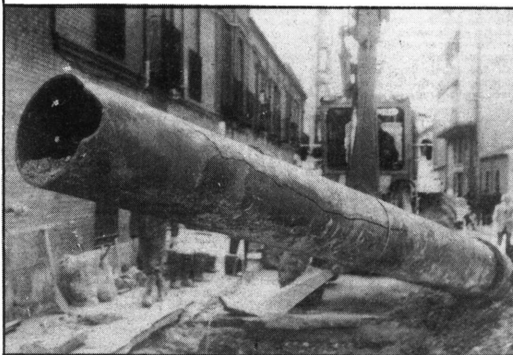
Una enorme grieta apareció en el tubo de hierro, de quinientos milímetros de diámetro, que forma parte de una de las principales arterias.—(Foto Cacho)
