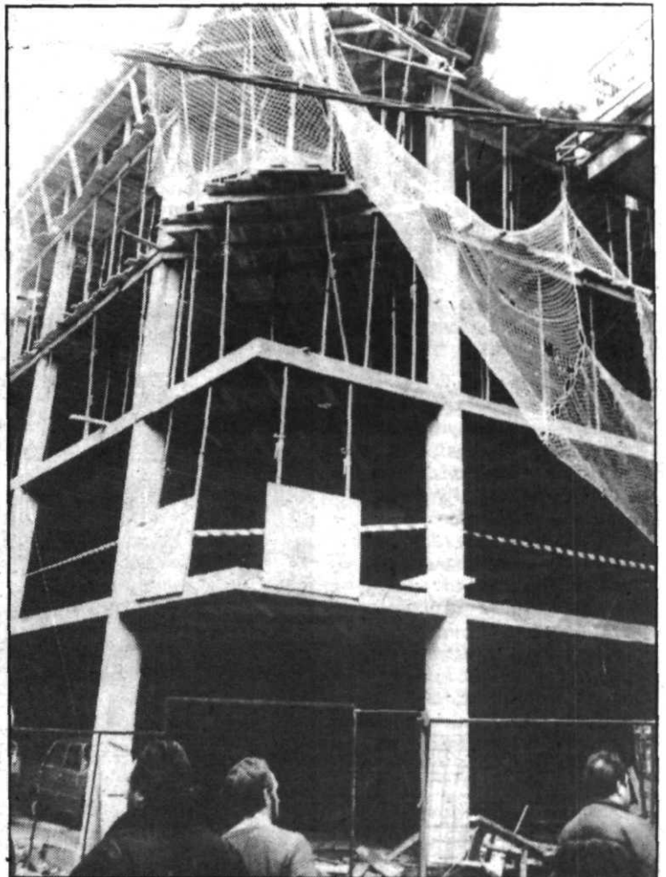
El derrumbamiento de un encofrado de hormigón en la cuarta planta de un piso en construcción ocasionó el trágico siniestro. (FOTOS WIFREDO)
